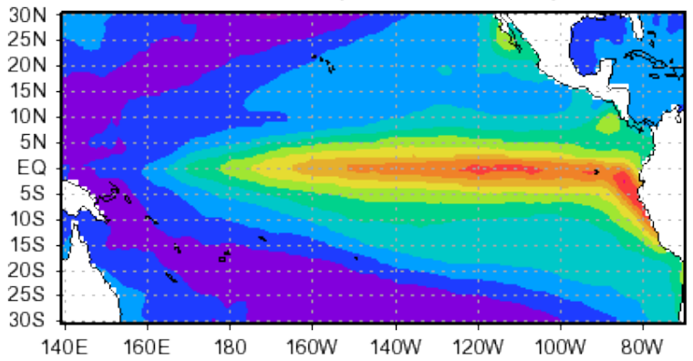
EOF 1 (42. % Var)
