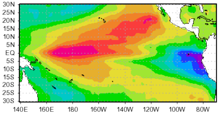
EOF 2 (11. % Var)
