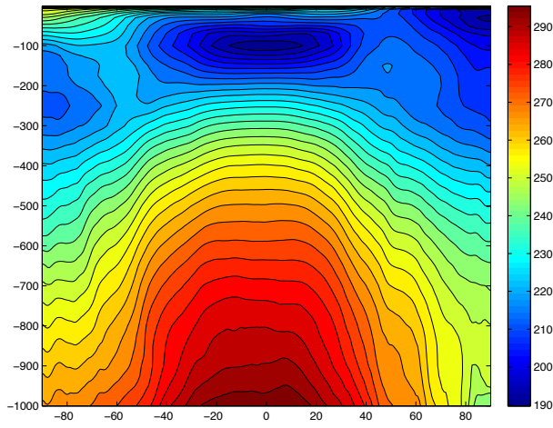
Figure 25 : moyenne zonale de la température le 25 décembre 1999.
