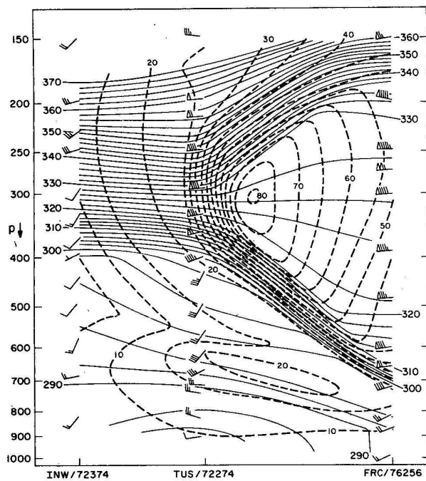
Figure 27 : Cross section à 0h GMT le 17 avril 1976 de la température potentielle (en K, traits continus) et de la vitesse du vent (en m/s, tirets).
