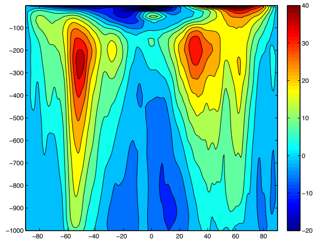
Figure 26: moyenne zonale du vent zonal.
