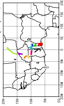
Ballons laches a J+12 h (04/05, 12 UTC)
