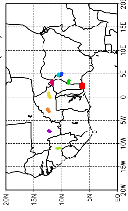
Ballons laches a J+30 h (09/05, 6 UTC)
