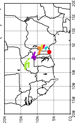
Ballons laches a J+84 h (11/05, 12 UTC)
