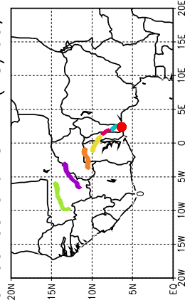
Ballons laches a J+84 h (18/05, 12 UTC)
