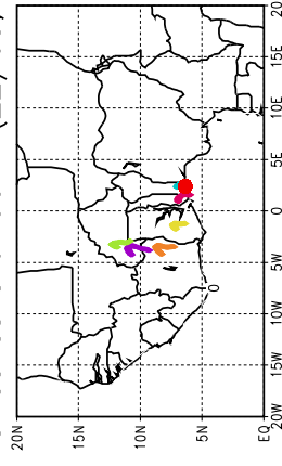
Ballons laches a J+90 h (22/05, 6 UTC)
