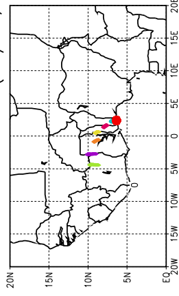
Ballons laches a J+90 h (28/05, 6 UTC)
