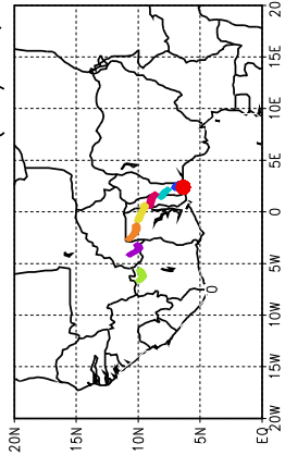
Ballons laches a J+66 h (27/05, 18 UTC)
