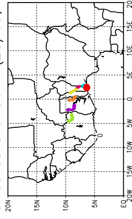
Ballons laches a J+90 h (28/05, 18 UTC)
