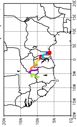
Ballons laches a J+60 h (27/05, 12 UTC)
