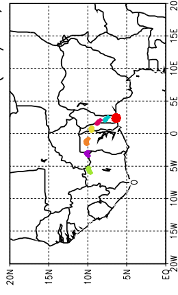
Ballons laches a J+78 h (28/05, 6 UTC)
