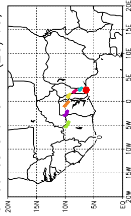
Ballons laches a J+84 h (28/05, 12 UTC)
