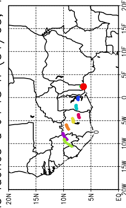
Ballons laches a J+48 h (31/05, 12 UTC)
