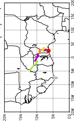
Ballons laches a J+90 h (08/06, 18 UTC)
