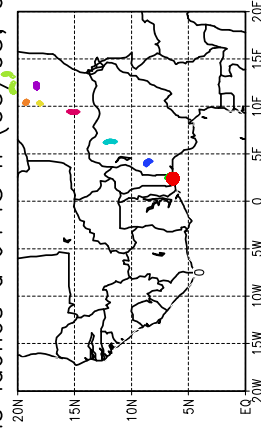
Ballons laches a J+48 h (03/05, 00 UTC)
