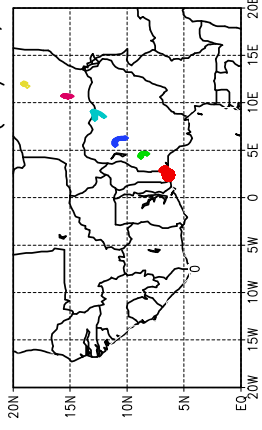
Ballons laches a J+18 h (13/05, 18 UTC)
