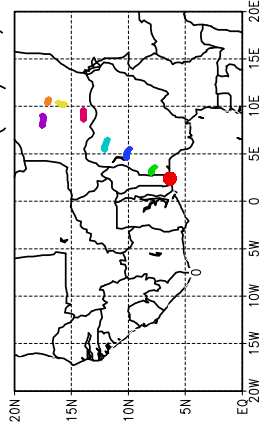
Ballons laches a J+36 h (14/05, 12 UTC)
