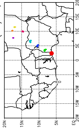
Ballons laches a J+30 h (14/05, 6 UTC)
