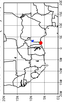
Ballons laches a J+48 h (17/05, 12 UTC)
