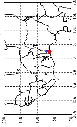
Ballons laches a J+66 h (18/05, 6 UTC)
