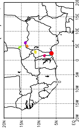
Ballons laches a J+66 h (22/05, 18 UTC)
