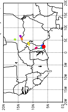
Ballons laches a J+60 h (22/05, 12 UTC)
