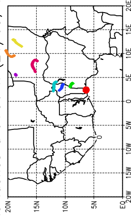
Ballons laches a J+36 h (21/05, 12 UTC)
