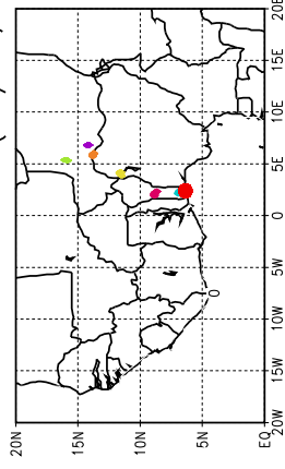
Ballons laches a J+90 h (23/05, 18 UTC)
