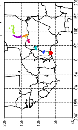
Ballons laches a J+42 h (23/05, 6 UTC)
