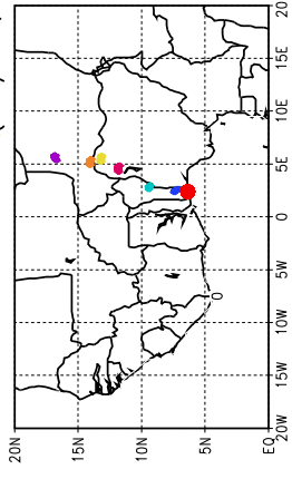
Ballons laches a J+66 h (24/05, 6 UTC)
