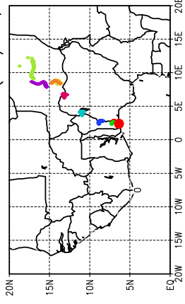
Ballons laches a J+18 h (22/05, 6 UTC)
