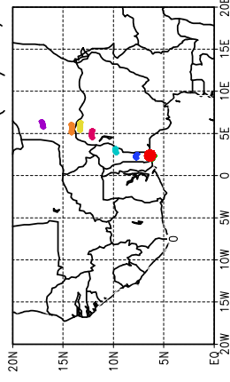
Ballons laches a J+30 h (22/05, 18 UTC)
