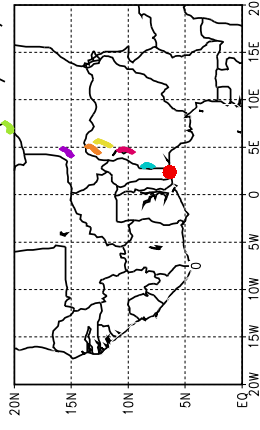
Ballons laches a J+78 h (24/05, 18 UTC)
