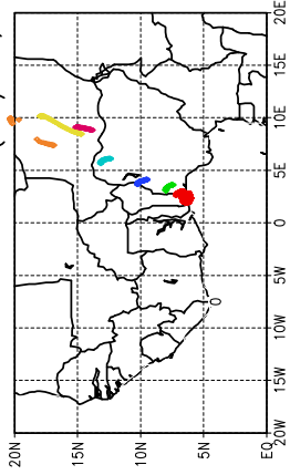
Ballons laches a J+12 h (22/05, 12 UTC)
