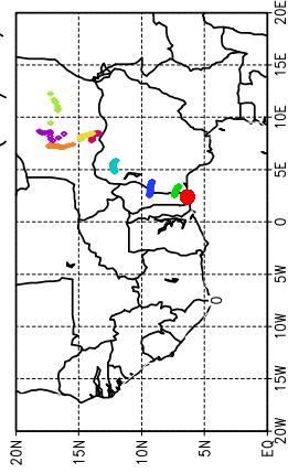
Ballons laches a J+36 h (23/05, 12 UTC)
