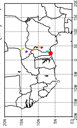
Ballons laches a J+84 h (25/05, 12 UTC)
