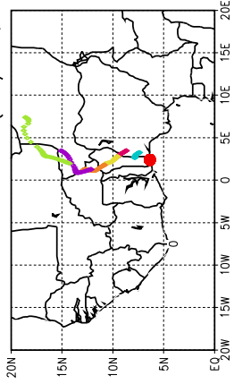
Ballons laches a J+84 h (28/05, 12 UTC)
