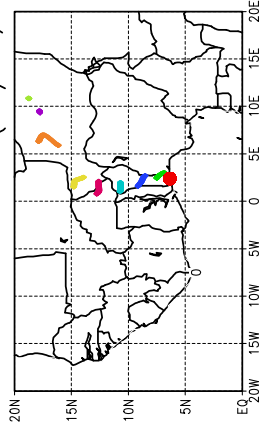
Ballons laches a J+36 h (27/05, 12 UTC)
