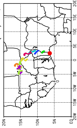
Ballons laches a J+36 h (08/06, 12 UTC)
