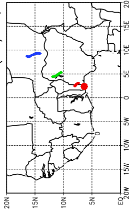
Ballons laches a J+18 h (08/05, 18 UTC)
