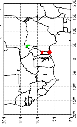
Ballons laches a J+12 h (08/05, 12 UTC)
