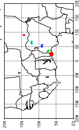
Ballons laches a J+36 h (13/05, 12 UTC)
