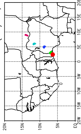
Ballons laches a J+42 h (13/05, 18 UTC)
