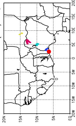
Ballons laches a J+66 h (14/05, 18 UTC)
