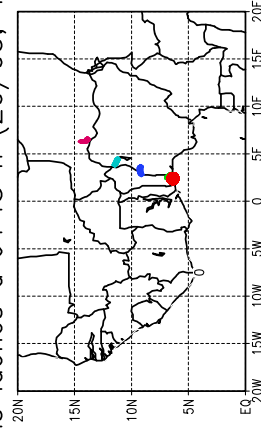
Ballons laches a J+48 h (20/05, 12 UTC)
