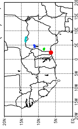
Ballons laches a J+30 h (19/05, 18 UTC)
