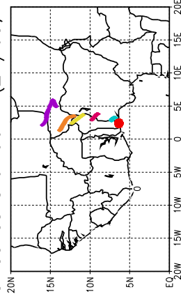
Ballons laches a J+90 h (27/05, 18 UTC)
