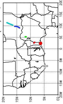
Ballons laches a J+12 h (24/05, 12 UTC)
