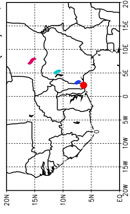
Ballons laches a J+66 h (03/06, 6 UTC)
