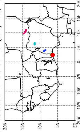
Ballons laches a J+48 h (24/06, 12 UTC)
