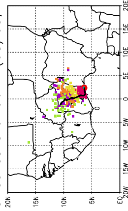
Ballons laches a J+96 h (08/05, 12 UTC)
