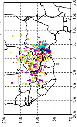
Ballons laches a J+66 h (20/05, 6 UTC)
