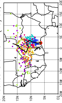
Ballons laches a J+48 h (19/05, 12 UTC)
