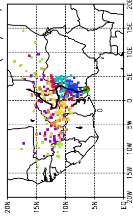
Ballons laches a J+42 h (19/05, 6 UTC)
