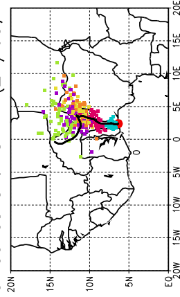
Ballons laches a J+84 h (24/05, 12 UTC)
