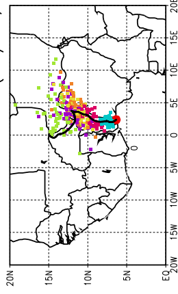
Ballons laches a J+78 h (24/05, 6 UTC)
