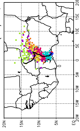
Ballons laches a J+66 h (23/05, 18 UTC)
