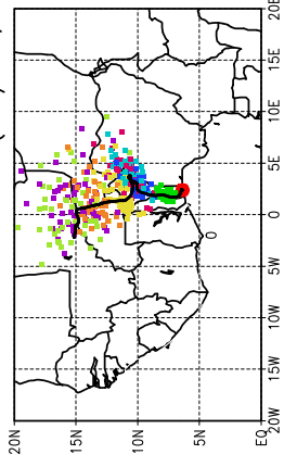
Ballons laches a J+18.h (23/05, 18 UTC)
