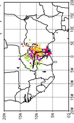
Ballons laches a J+90 h (27/05, 6 UTC)
