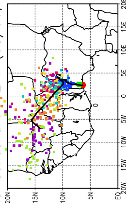
Ballons lâchés à J+42 h (08/06, 6 UTC)
