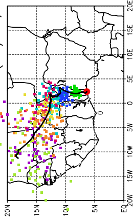
Ballons lâchés à J+24 h (07/06, 12 UTC)
