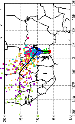
Ballons lâchés à J+36 h (08/06, 00 UTC)
