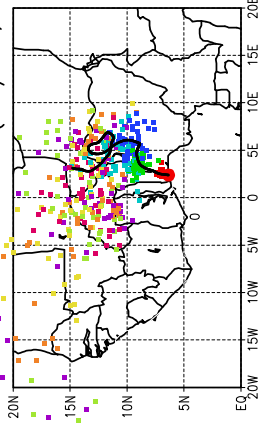
Ballons lâchés à J+18 h (08/06, 18 UTC)
