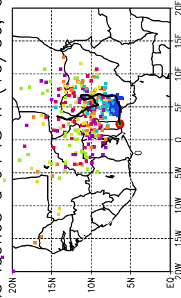
Ballons lâchés à J+48 h (10/06, 00 UTC)
