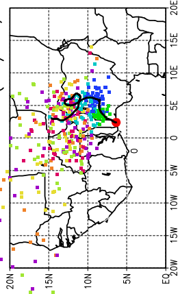
Ballons lâchés à J+24 h (09/06, 00 UTC)
