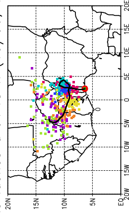
Ballons laches a J+48 h (19/06, 12 UTC)
