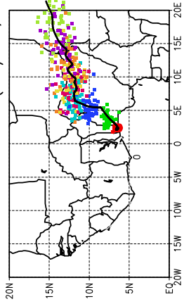
Ballons laches a J+12 h (28/06, 12 UTC)
