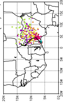
Ballons laches a J+90 h (13/07, 6 UTC)
