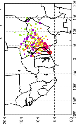
Ballons laches a J+96 h (13/07, 12 UTC)
