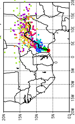
Ballons laches a J+30 h (13/07, 18 UTC)
