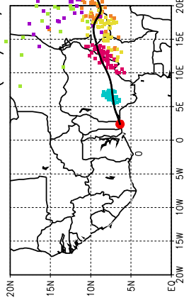
Ballons laches a J+78 h (20/07, 6 UTC)
