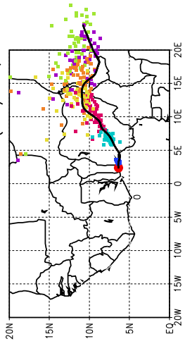
Ballons laches a J+66 h (23/07, 18 UTC)
