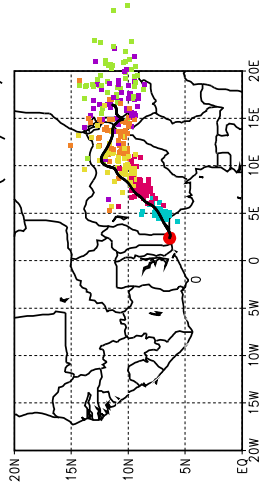
Ballons laches a J+78 h (24/07, 6 UTC)
