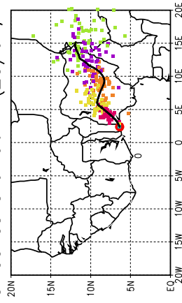
Ballons laches a J+96 h (25/07, 12 UTC)
