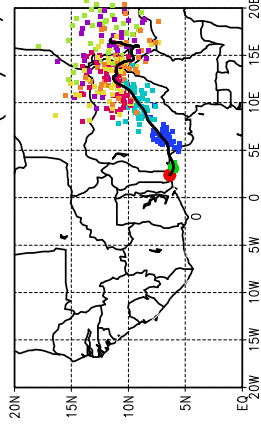
Ballons laches a J+42 h (23/07, 6 UTC)
