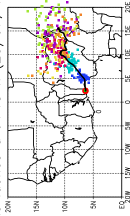
Ballons laches a J+48 h (23/07, 12 UTC)
