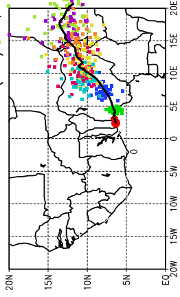
Ballons laches a J+18 h (23/07, 6 UTC)
