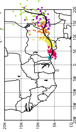
Ballons laches a J+90 h (27/07, 6 UTC)
