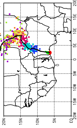
Ballons laches à J+42 h (12/05, 6 UTC)
