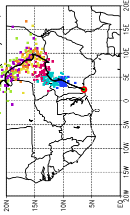
Ballons laches à J+48 h (12/05, 12 UTC)
