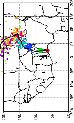
Ballons laches à J+30 h (11/05, 18 UTC)
