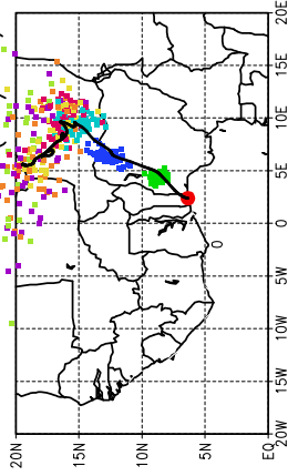
Ballons laches a J+24 h (13/05, 12 UTC)
