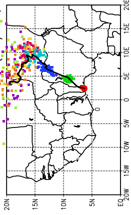
Ballons laches a J+18 h (13/05, 6 UTC)
