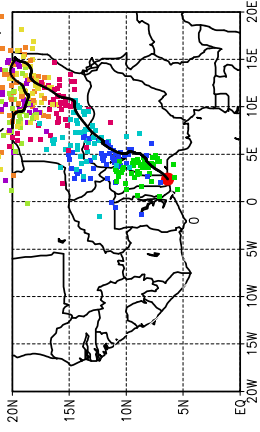
Ballons laches a J+30 h (20/05, 18 UTC)
