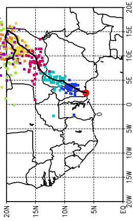
Ballons laches a J+48 h (21/05, 12 UTC)
