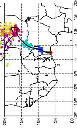
Ballons laches a J+12 (22/05, 6 UTC)
