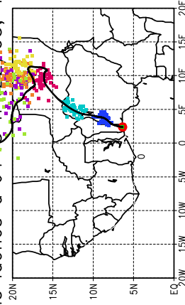
Ballons laches a J+14 (22/05, 12 UTC)
