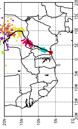
Ballons laches a J+78 h (23/05, 18 UTC)
