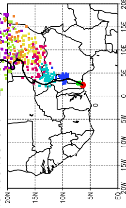
Ballons laches a J+42 h (27/05, 18 UTC)
