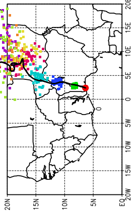
Ballons laches a J+30 h (27/05, 6 UTC)
