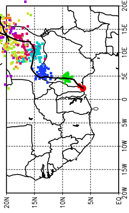
Ballons laches a J+18 h (27/05, 18 UTC)
