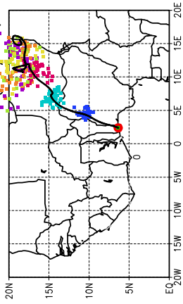
Ballons laches a J+48 h (30/06, 12 UTC)
