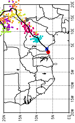
Ballons laches a J+66 h (03/07, 6 UTC)
