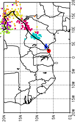
Ballons laches a J+66 h (03/07, 18 UTC)
