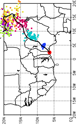
Ballons laches a J+60 h (03/07, 12 UTC)
